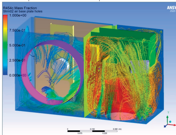
Dinámica de flujo computacional de la unidad condensadora Danfoss Optyma™.
