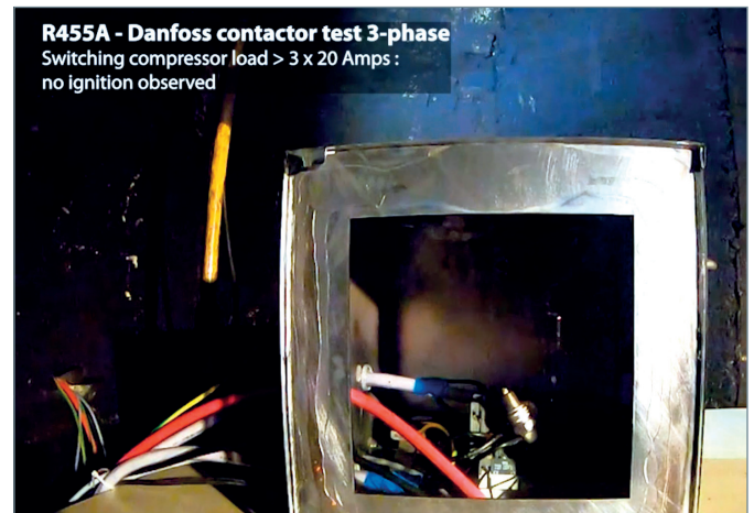
Prueba de ignición en laboratorio independiente.
